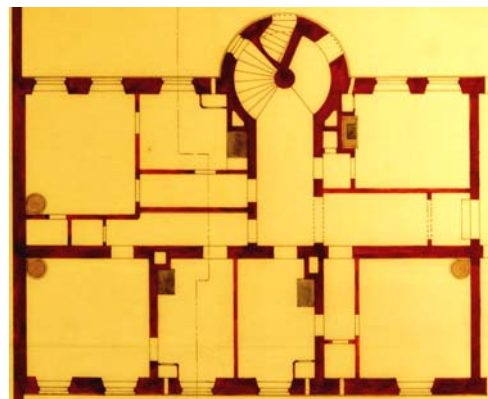
Gårdshusets bottenvåning enligt ritning 1894
