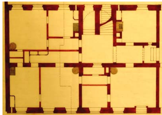
Gathusets bottenvåning enligt ritning 1894
